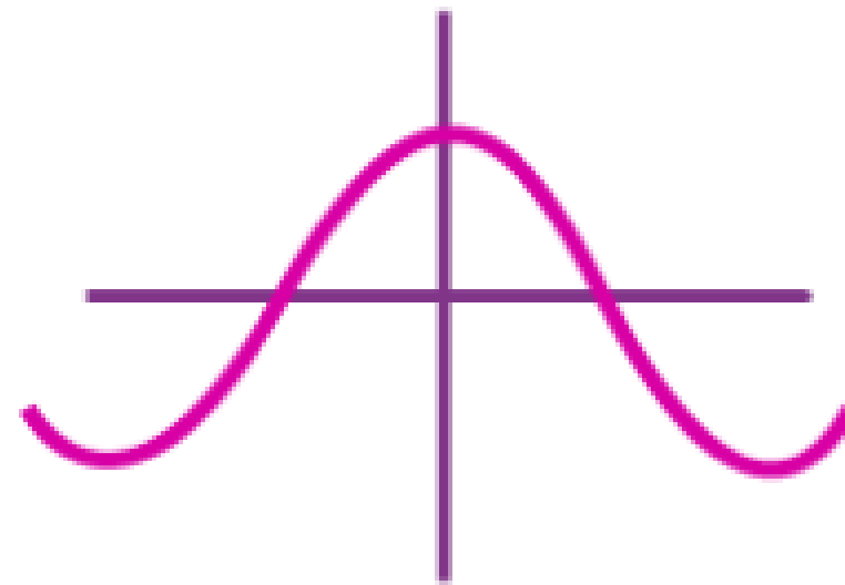
\cos x (even)
