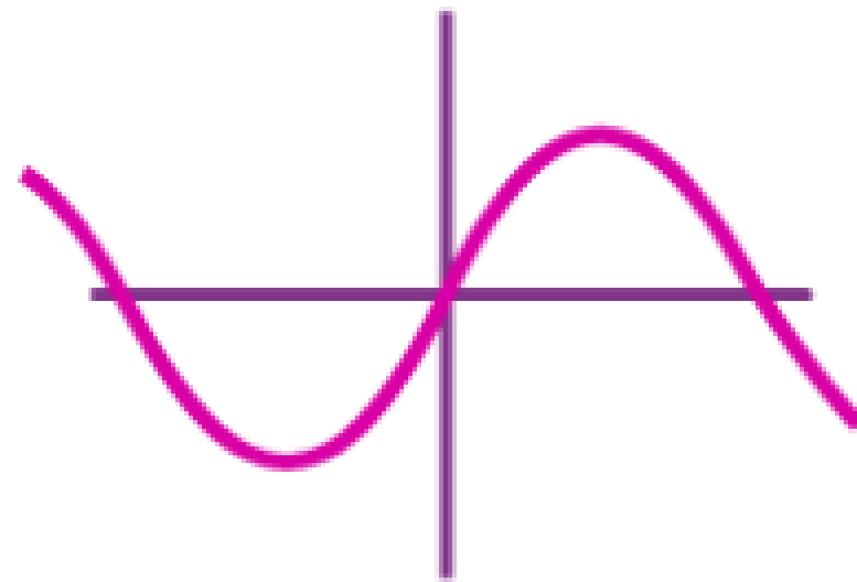
\sin x (odd)
